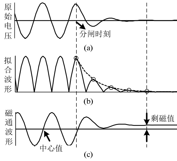
图 A.1 剩磁测算原理
