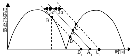
图 D. 3 关合系数 k < 1 时的关合特性曲线
