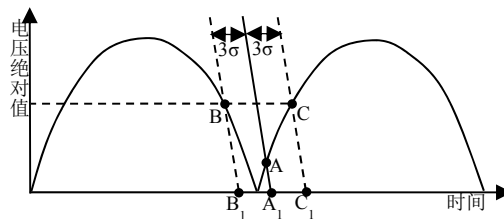
图 D. 2 关合系数 k \geq 1 时的关合特性曲线
