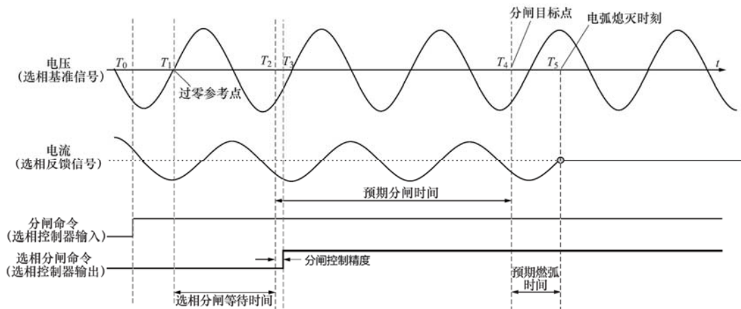
图 C.2 选相分闸控制示意图
