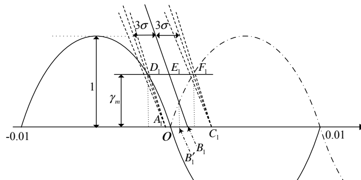
图 D.1 断路器 RDDS 及其分散性
