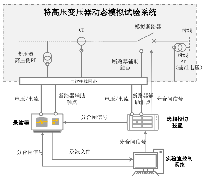
图 B.1 装置功能试验二次接线回路示意图
