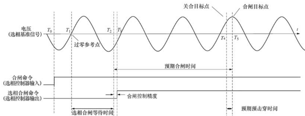
图 C.1 选相合闸控制示意图
