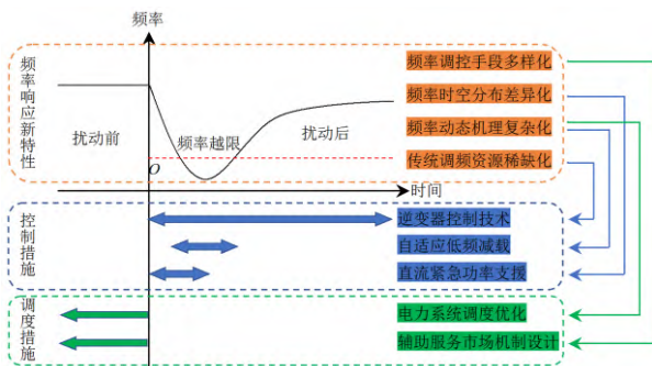
图 6 双高电力系统频率响应改善措施
