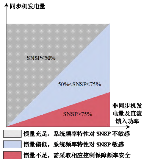
图5 SNSP对爱尔兰电网频率安全性的影响
