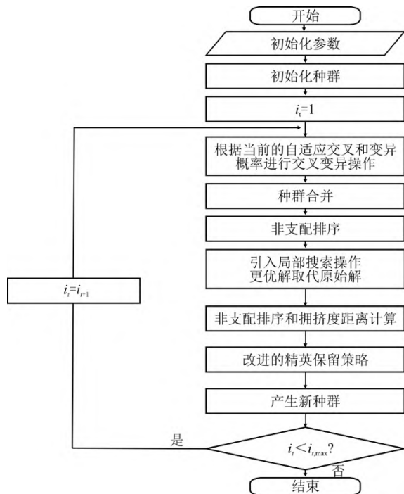
图 3 改进 NSGA-II 优化流程
