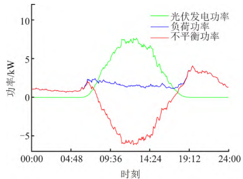
图 4 典型日光伏、负荷功率变化曲线
