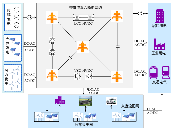
图 1 “双高”电力系统的结构示意图
