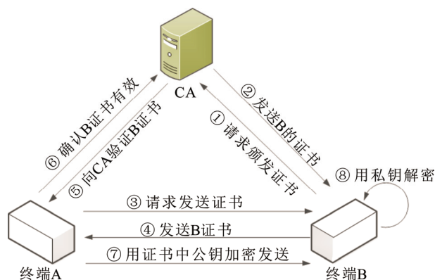
图 2 基于 PKI 体系的终端加密认证流程
