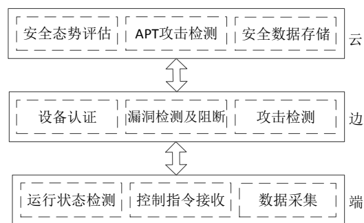
图3 边缘计算安全防护体系架构
