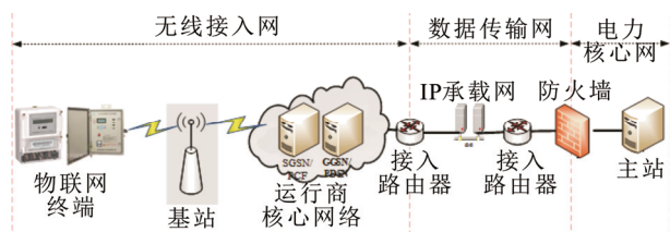
图5 电力无线虚拟专网
