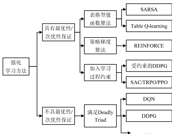
图3 根据性能保证对强化学习方法的分类
